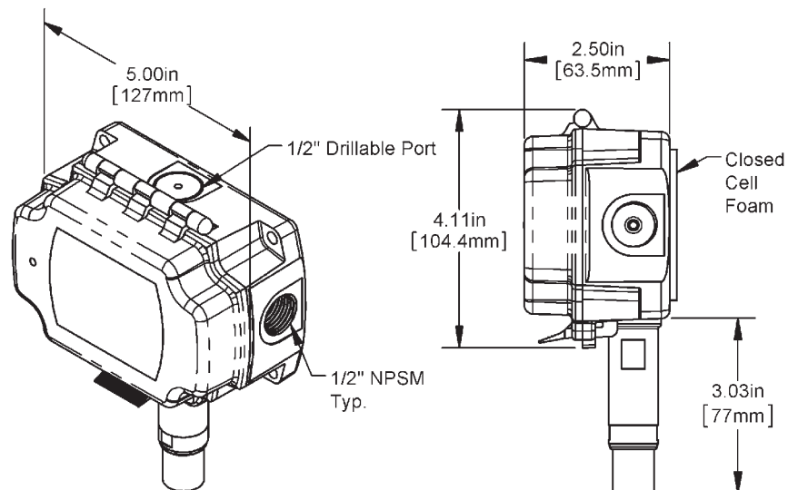
BAPI-Box (BB)
