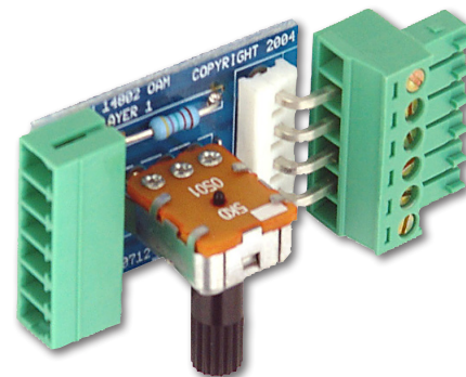
OAM - Output Adjust Module
