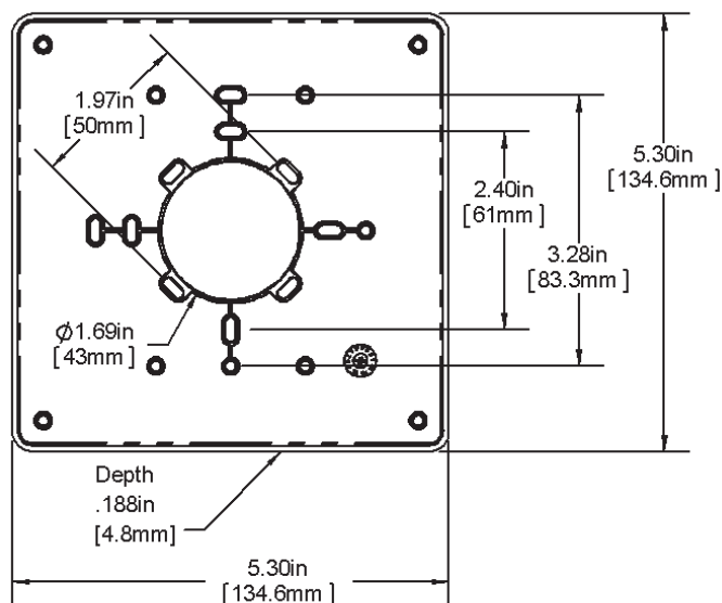
BA/ADP-53-53-BW
