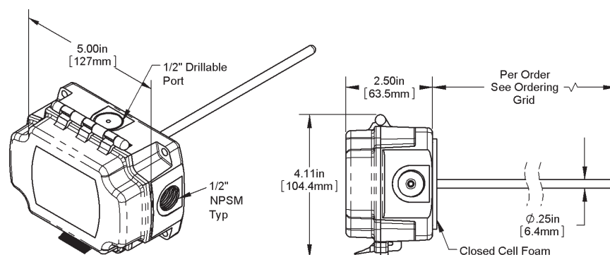
BAPI-Box (BB)
