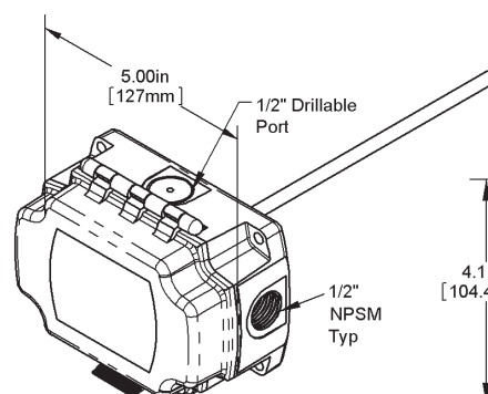
BAPI-Box (BB)
