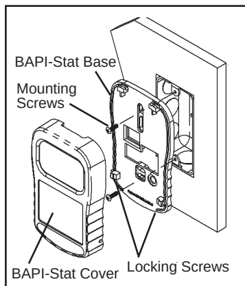
BAPI-Stat Style Enclosure
