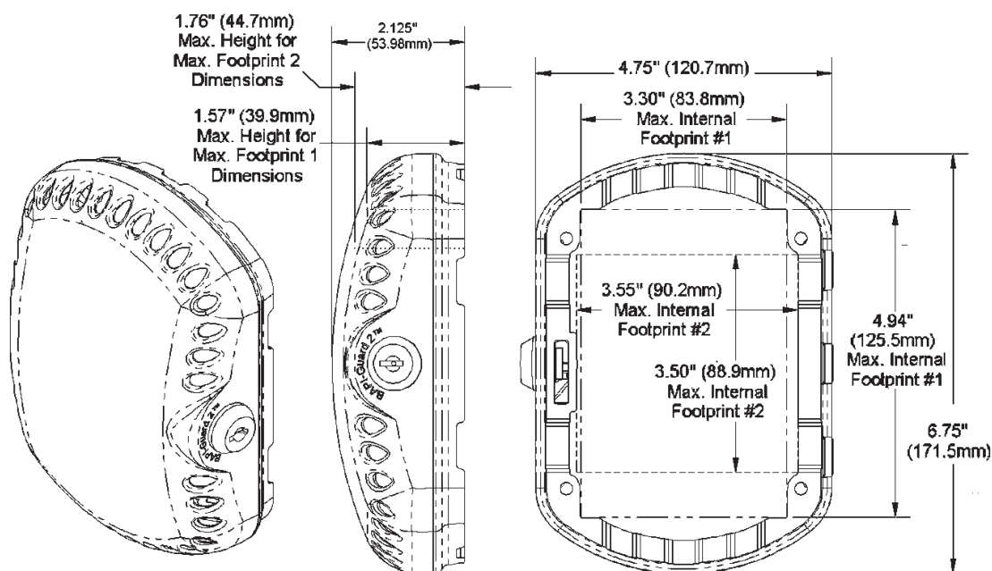
BAPI-Guard 2
