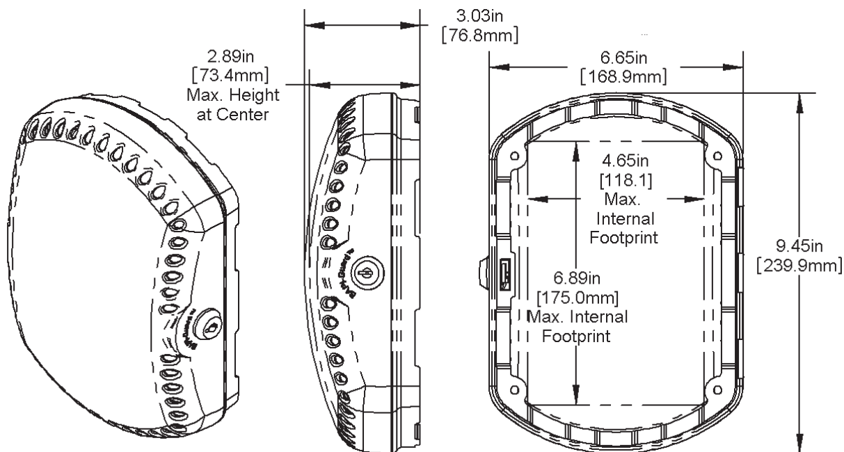
BAPI-Guard
